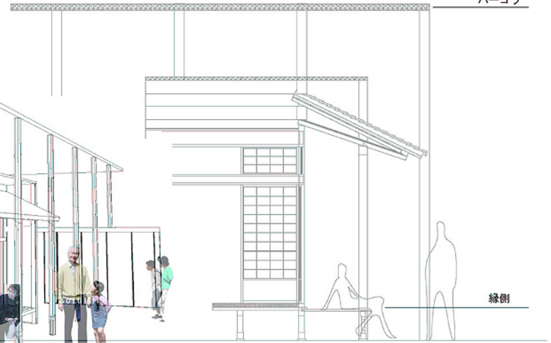
断面詳細図 scale: 1/25
