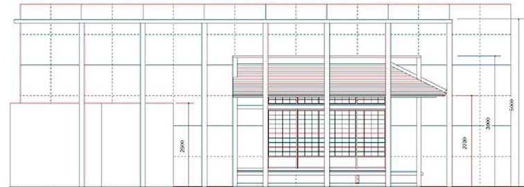
南側立面図 scale: 1/50
